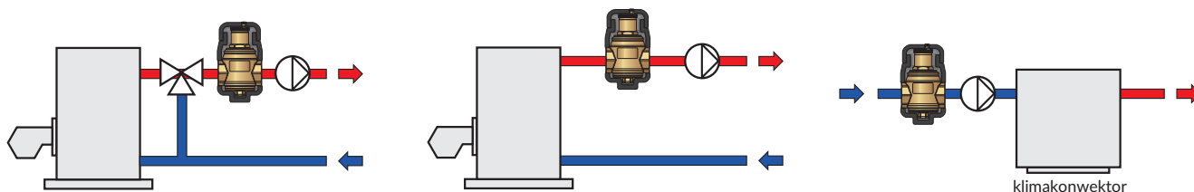
Rys. 20 Prawidłowy montaż:
