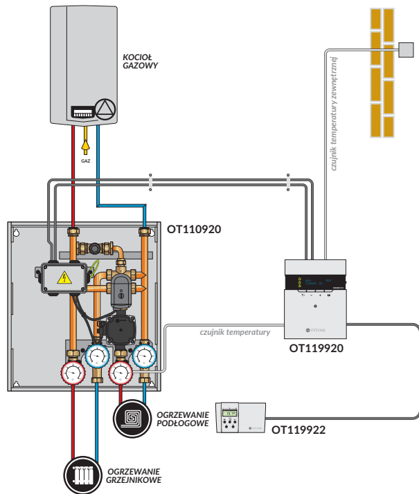
Rys. 29 Przykładowy schemat zastosowania - NOVACOND
