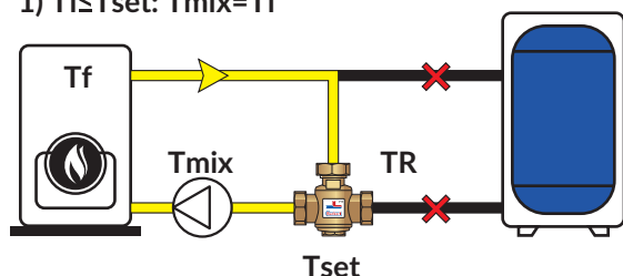
Rys. 13 Schemat działania
