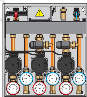
OT110907 sprzęgło-rozdzielacz
