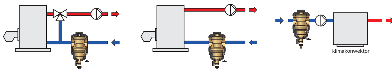
Rys. 12 Prawidłowy montaż:
