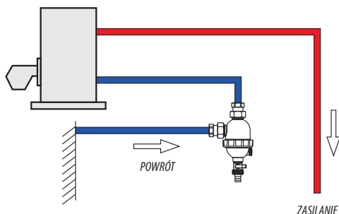
Rys. 10 Prawidłowy montaż: w systemach ogólnych
