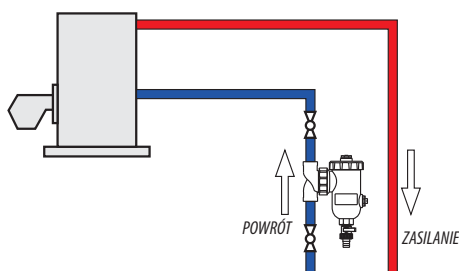
Rys. 11 Prawidłowy montaż: w systemach ogólnych
