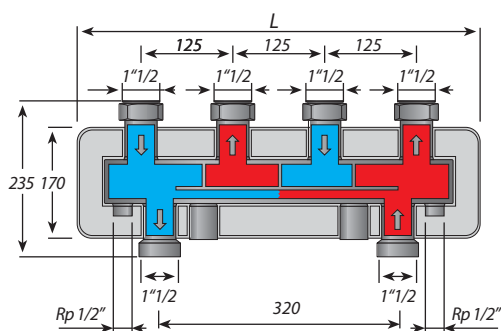
Rys. 42 Wymiary sprzęgło-rozdzielaczy
