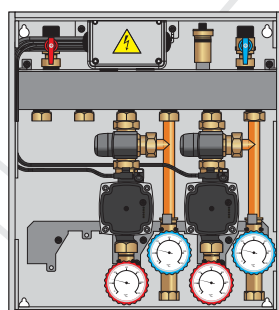
OT110911 sprzęgło-rozdzielacz
