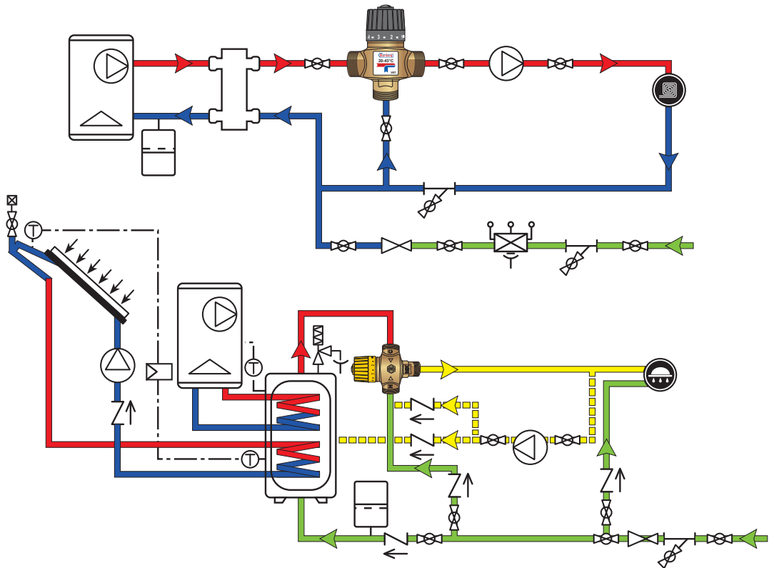
Rys. 16 Przykładowy schemat zastosowania mieszaczy termostatycznych
