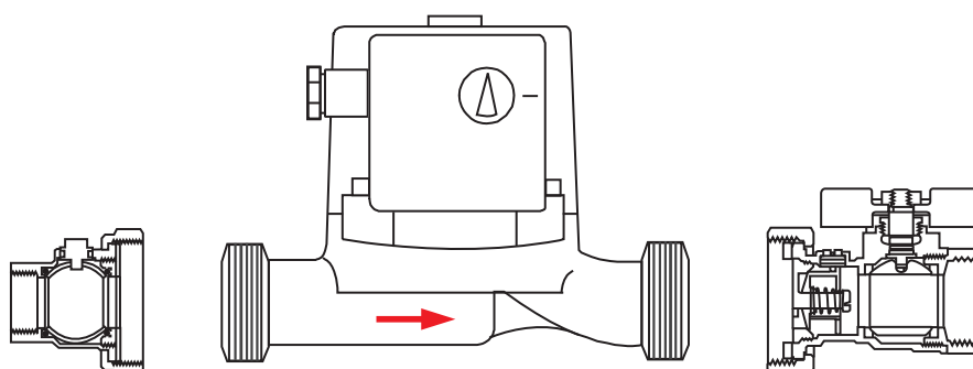
Rys. 19 Podłączenie pompy do instalacji z zastosowaniem zaworów OT0801
